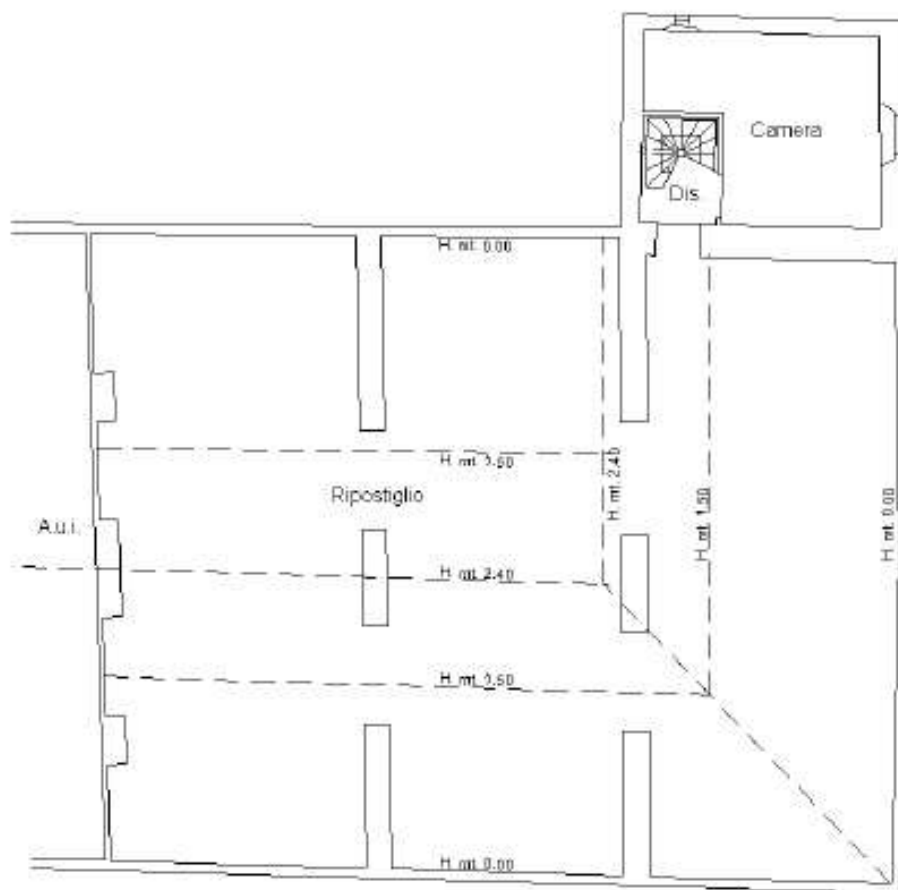
Piano Secondo - H. media mt. 1.20
