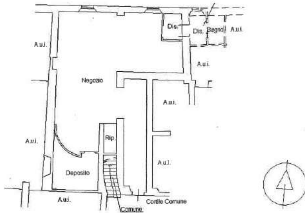
Piano Terra - H. mt. 2.70
